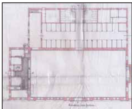
Manēžas un staļļa pirmā stāva plāns (1895., arh. K. Felsko).
